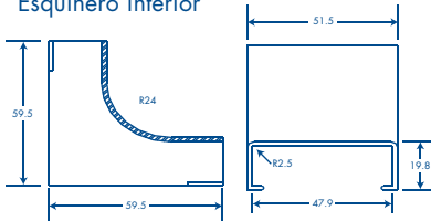
Pieza unión
