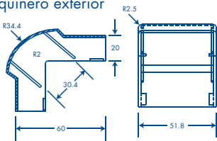
Esquinero exterior
