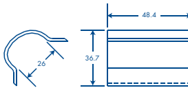
Esquinero interior
