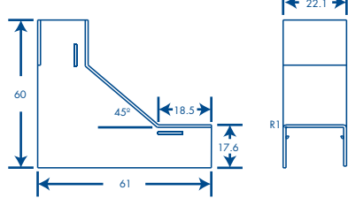
Esquinero interior
