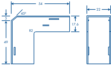
Esquinero exterior
