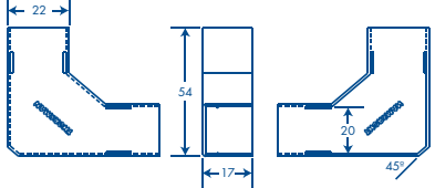
Sección T
