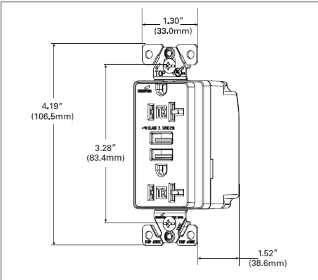
Figura 2. Dimensiones TR7756
