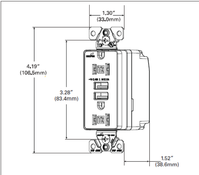
Figura 1. Dimensiones TR7755
